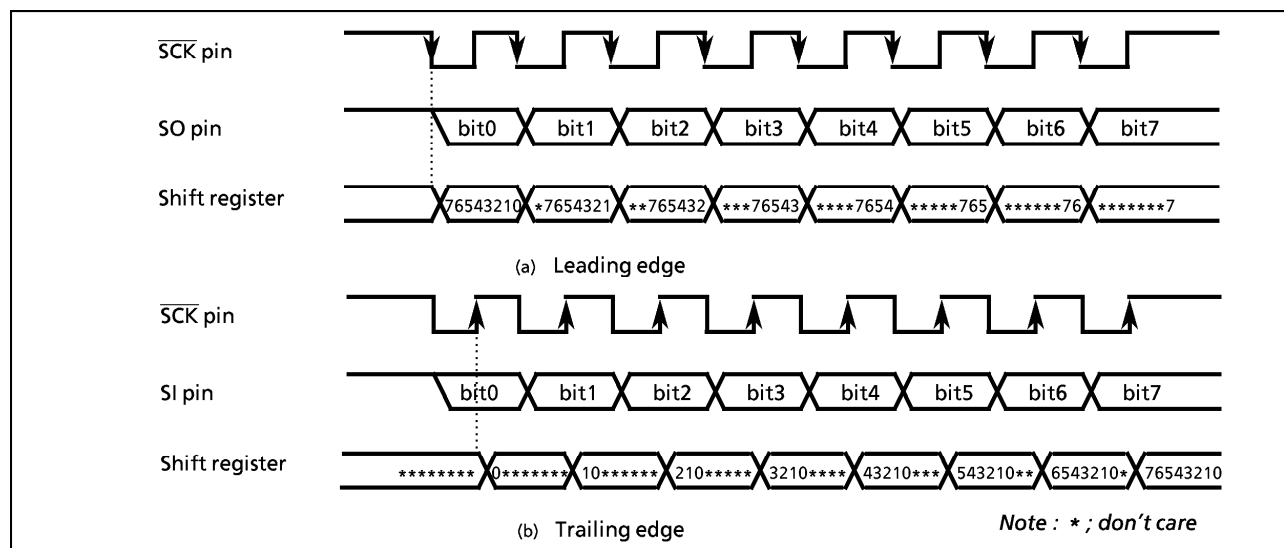
Figure 2-44. Shift Edge
