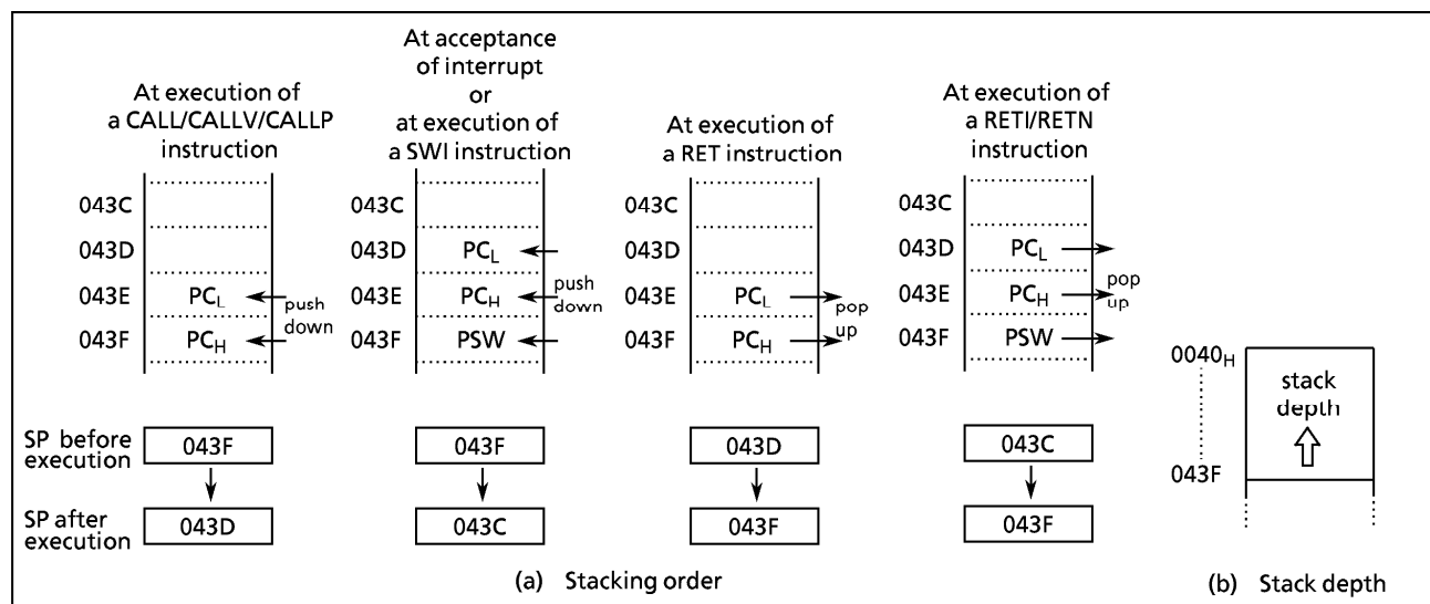
Figure 1-8. Stack
