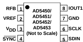
TSOT (UJ-8)
