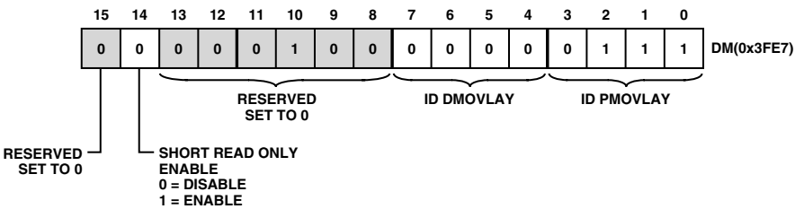
a. IDMA Overlay
