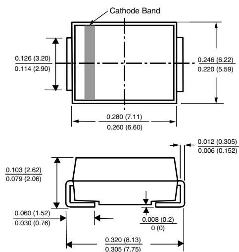
DO-214AB (SMCJ)
