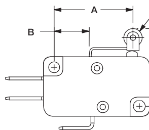
FIG. 1 Lever Roller
