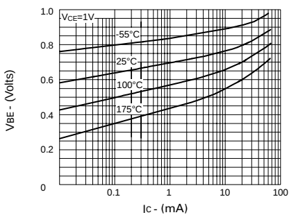
V_{BE(on)} v I_C
