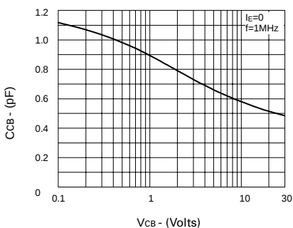
C_{CB} v V_{CB}
