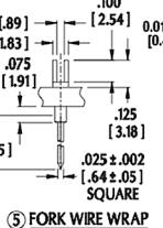
⑤ FORK WIRE WRAP
