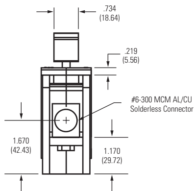
Solderless Connector (- F0)
