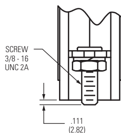
Stud (-B3)
