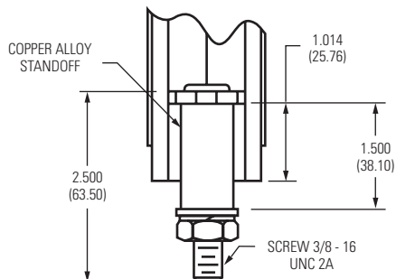
Long Stud (-B4)
