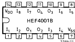
Fig. 2 Pinning diagram.
