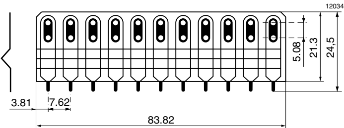
Fig. 14 H11 Flexi-PCB
