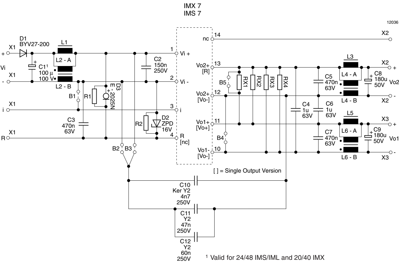
Fig. 9a C/DMB IMX/S 7 circuit diagram
