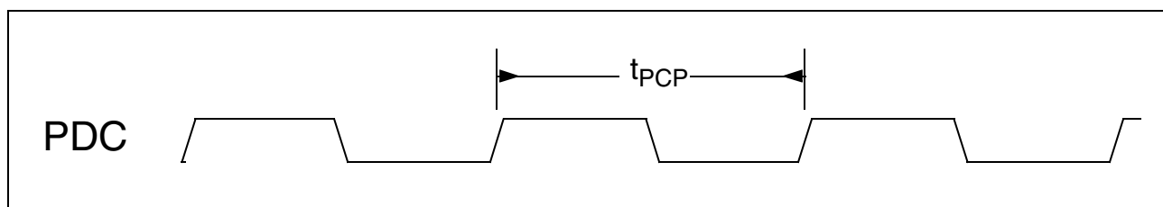
Figure 79 PDC Parameters
