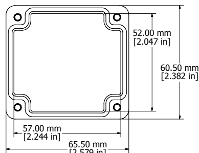
LID - INSIDE
