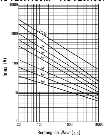
ROV20H820K – ROV20H511K
