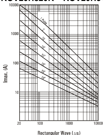
ROV20H820K – ROV20H511K
