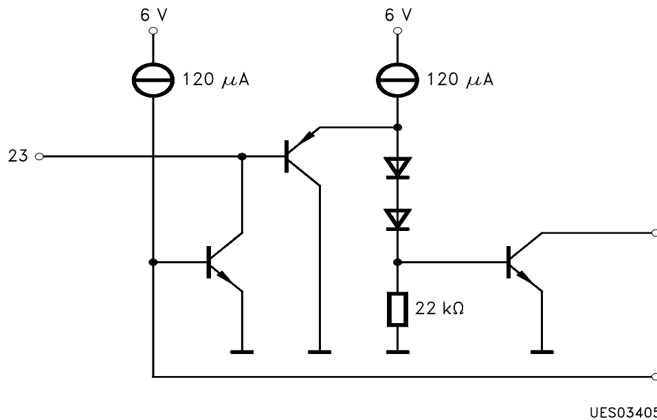
I²C Bus SDA (Pin 23)
