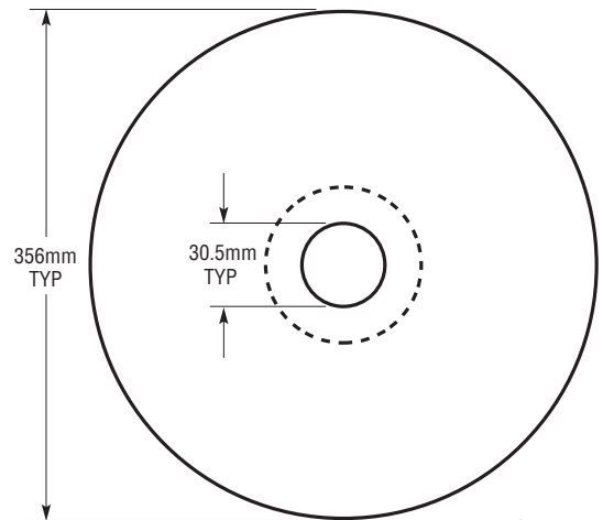
TO-92 Reel Dimensions
