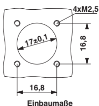
Einbaumaße
