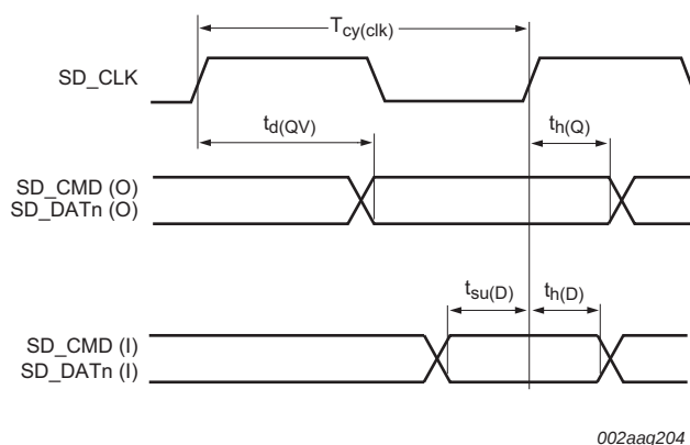
Fig 30. SD/MMC timing
