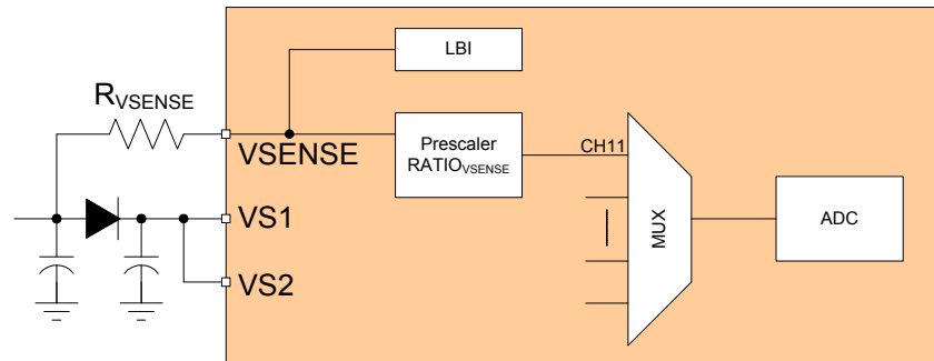
Figure 42. VSENSE Module
