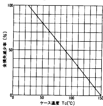
全損失減少率—ケース温度 Power Derating
