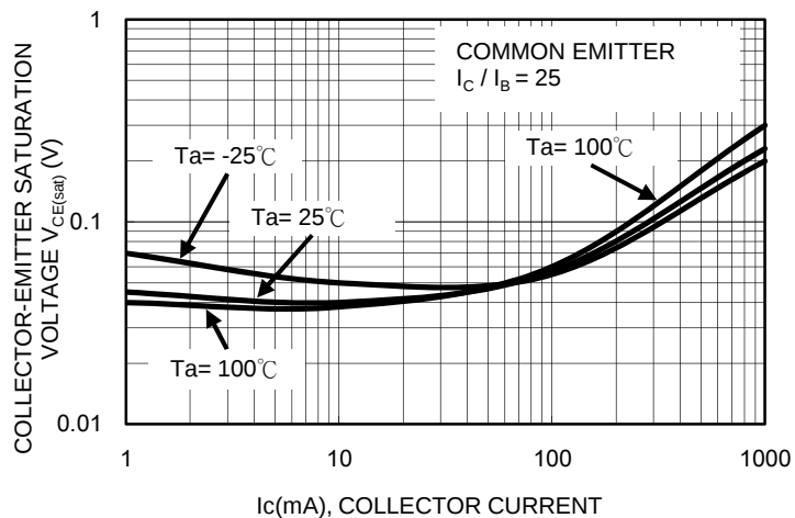
FIG. 6 V_{ce(sat)} - I_c
