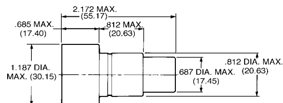
Receptacle
