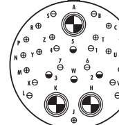
24-20 10#20 13#16 4#12 3 TWINAX #8 (N)
