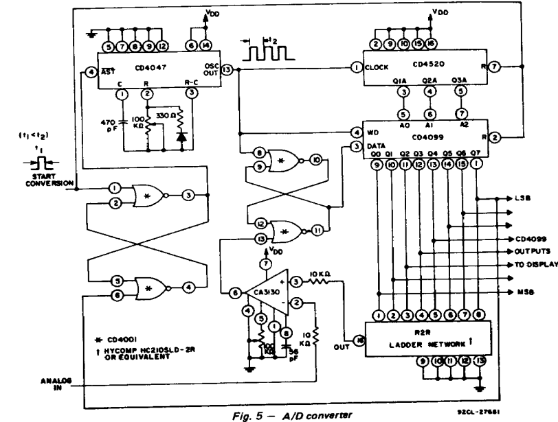
Fig. 5 - A/D converter
