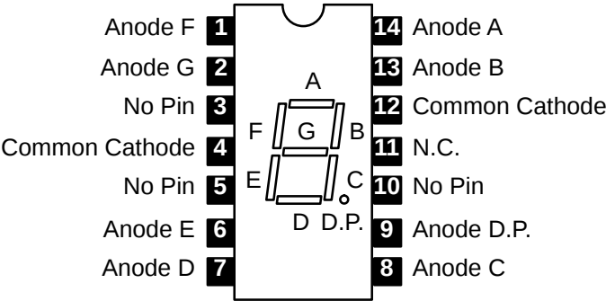
NTE3069, NTE3071
