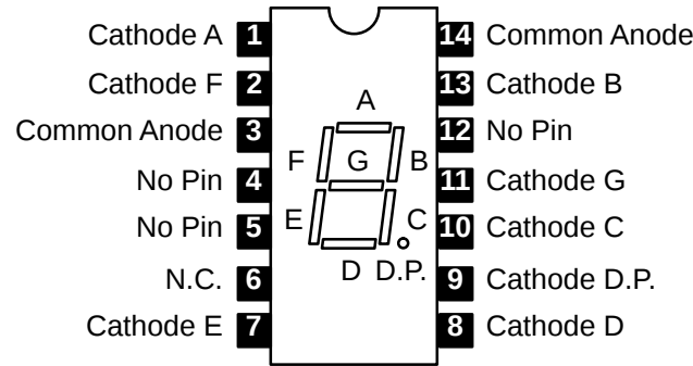
NTE3068, NTE3070
