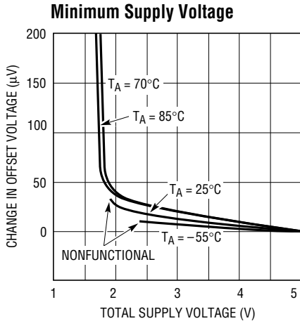
LT1366 TPC10
