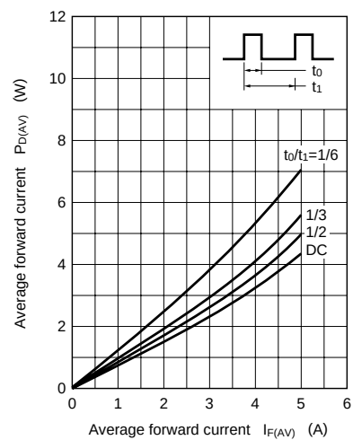
P_{D(AV)} - I_{F(AV)}
