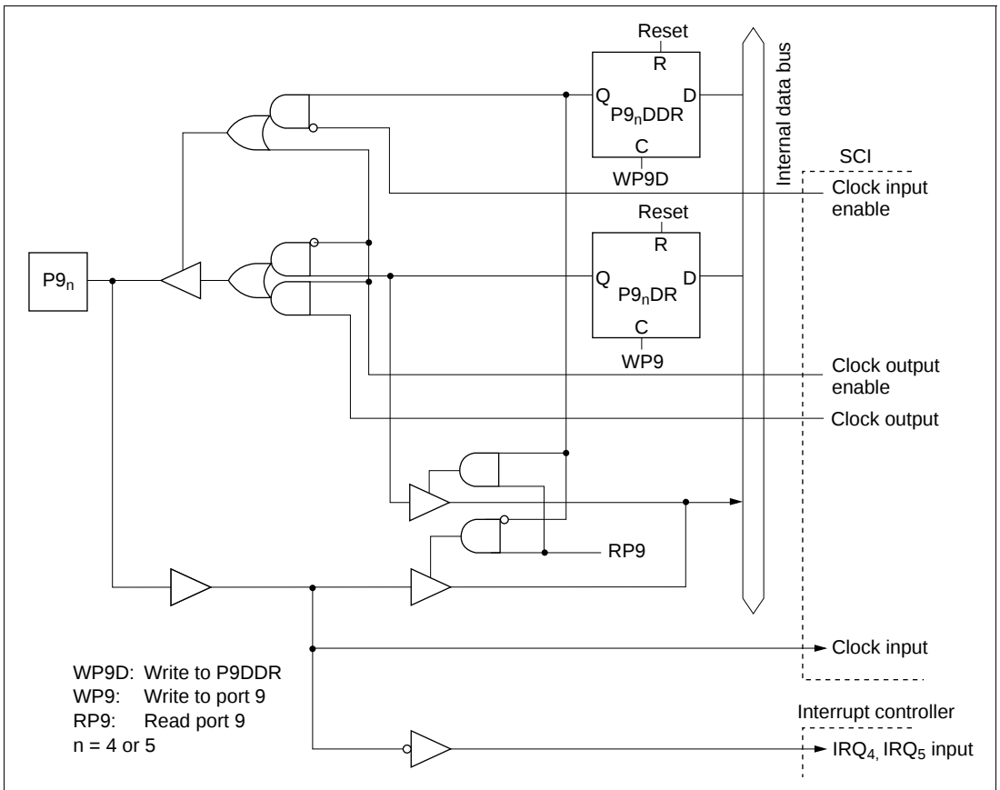
Figure C-8 (d) Port 9 Block Diagram (Pins P9 4 and P9 5 )
