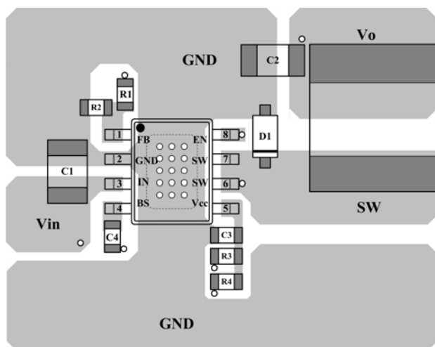
Top Layer
