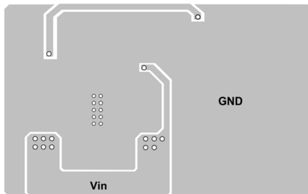
Bottom Layer
