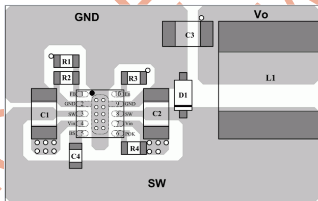
Top Layer
