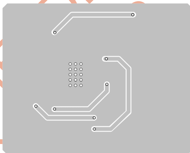
Bottom Layer
