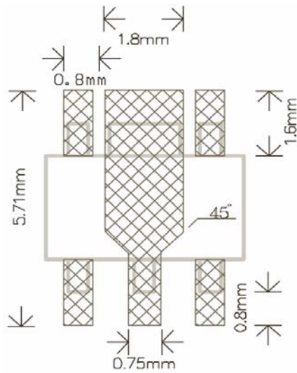
SOT-89-5
