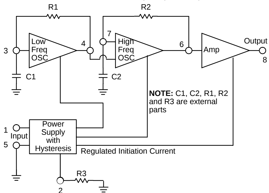
Pin Connection Diagram (NTE1649)
