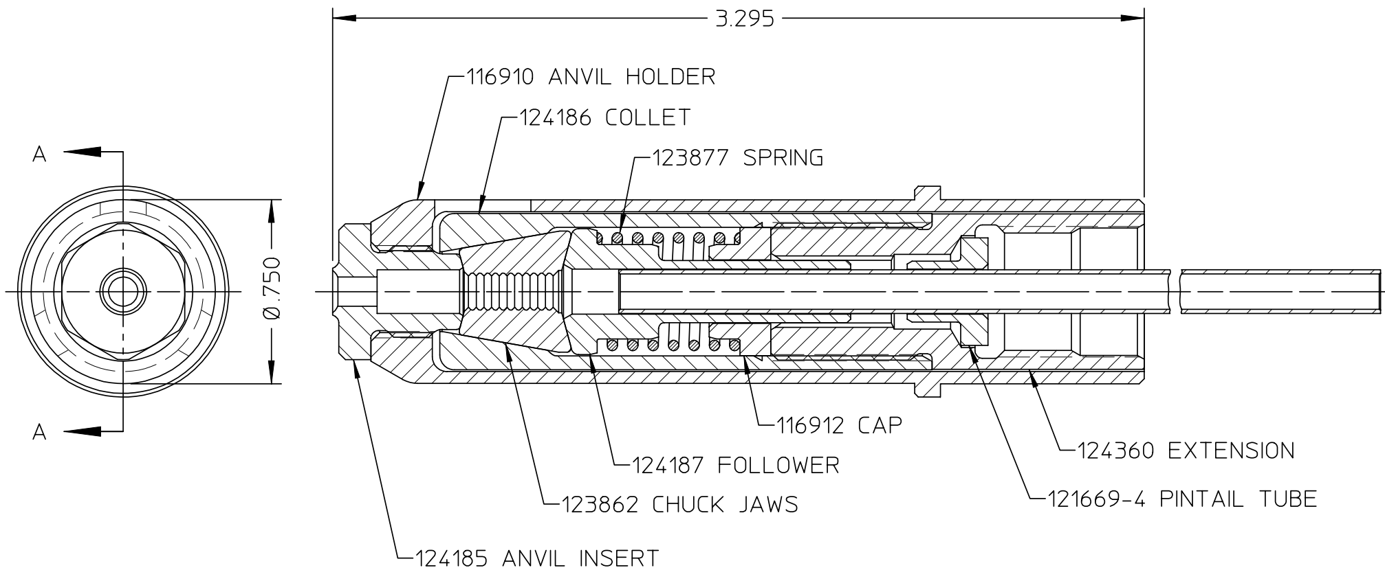
SECTION A-A
