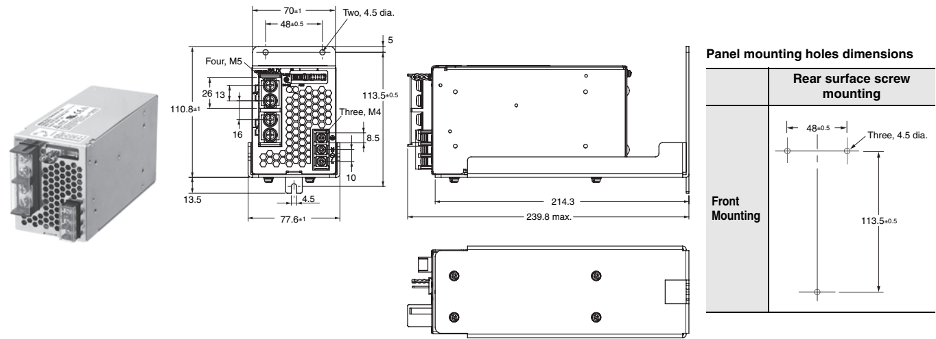
S8JX-P300□□C (300 W)
