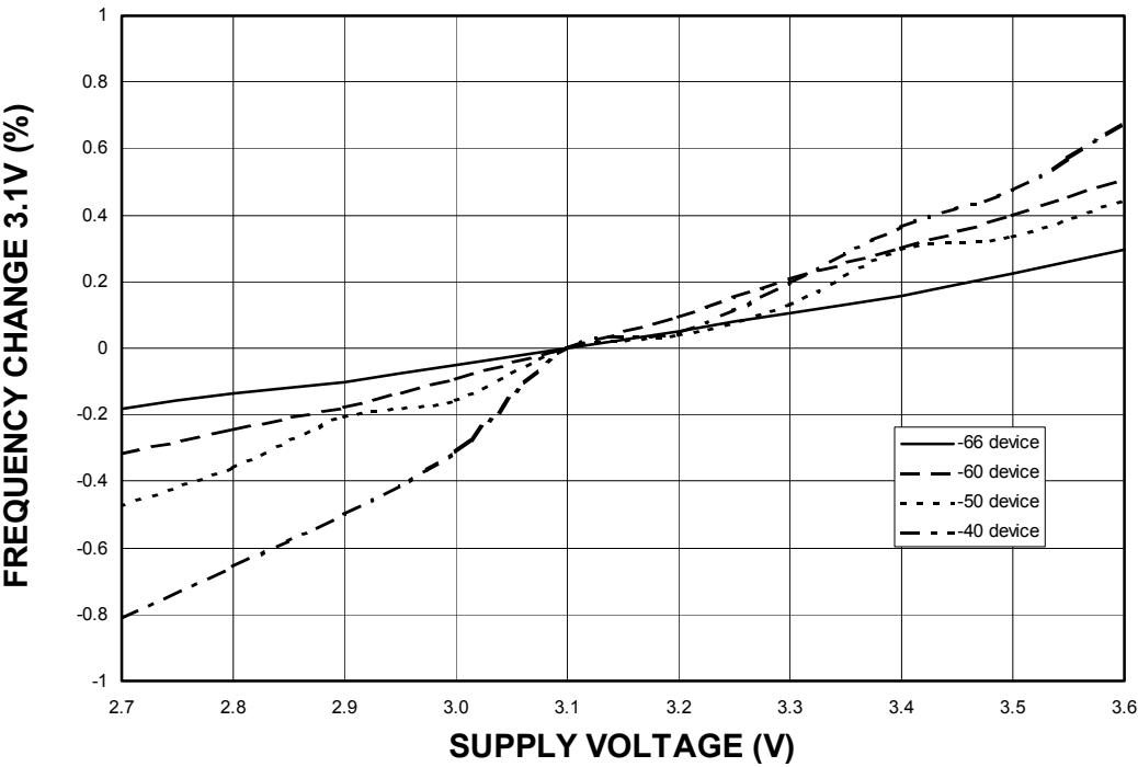
DS1077L VOLTCO
