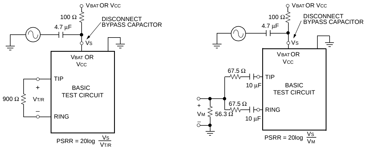
Figure 7. Longitudinal PSRR
