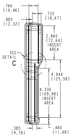
SECTION A-A
