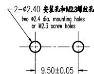
安装孔图 Mounting Holes
