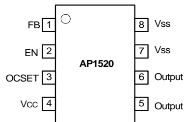
SO-8
