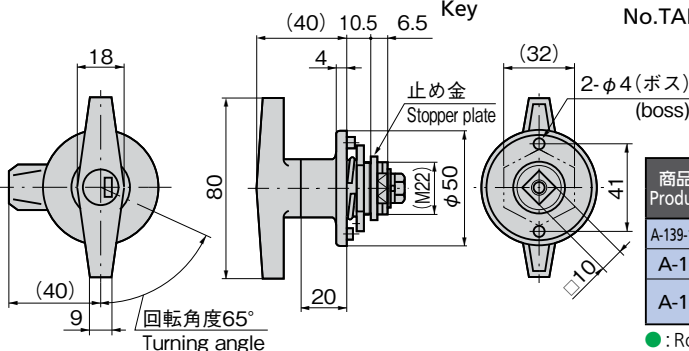
キーNo.0200 Key
