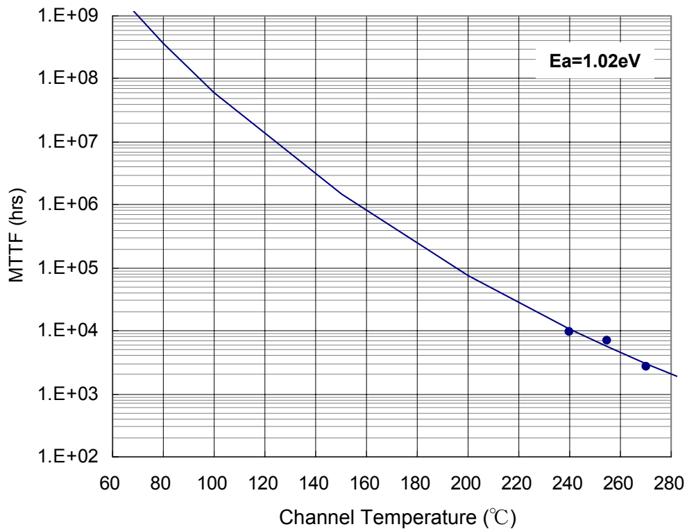
MTTF vs \Delta T_{ch}
