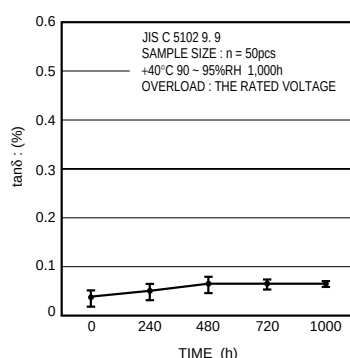
Fig.26 tanδ
