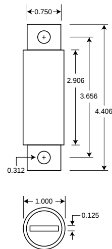
Fig. 2: 70-100 Amp Range
