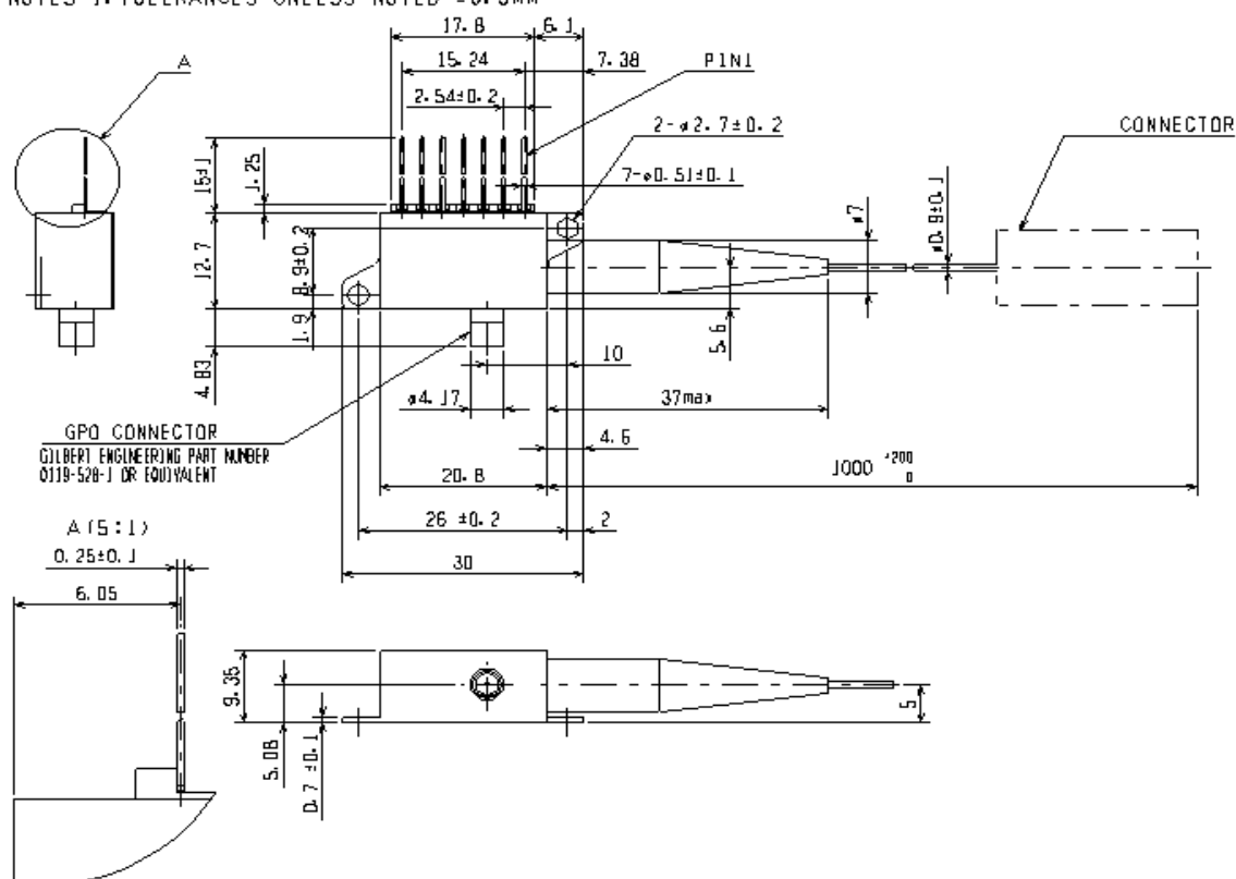
FU-653SEA-2Mxx/3Mxx
