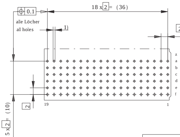
Lochbild für Leiterplatte (Bestückungsseite)
