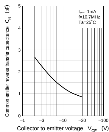
C_{re} - V_{CE}
