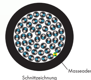
Schnittzeichnung
