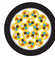
Schnittzeichnung
