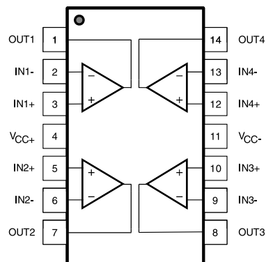
TSSOP14
