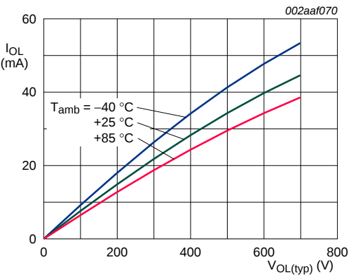
b. V_{DD(I/O)0} or V_{DD(I/O)1} = 2.6\text{ V}
