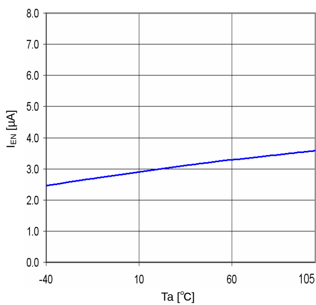
Fig.24 T_a - I_{EN}
