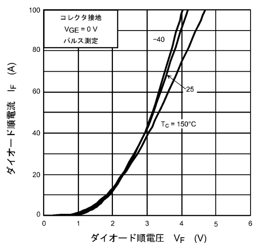
図 8.10 I_F - V_F
