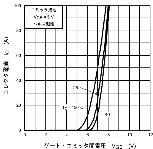
図 8.5 I_C - V_{GE}
