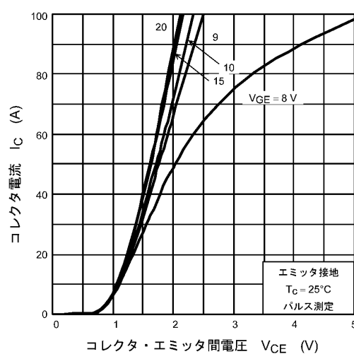
図 8.2 I_C - V_{CE}
