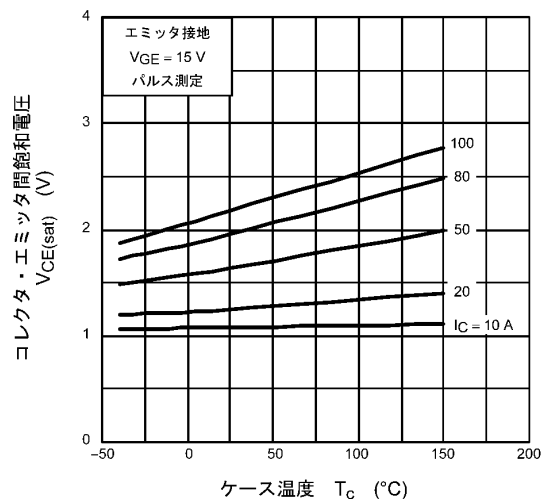
図 8.4 V_{CE(sat)} - T_C
