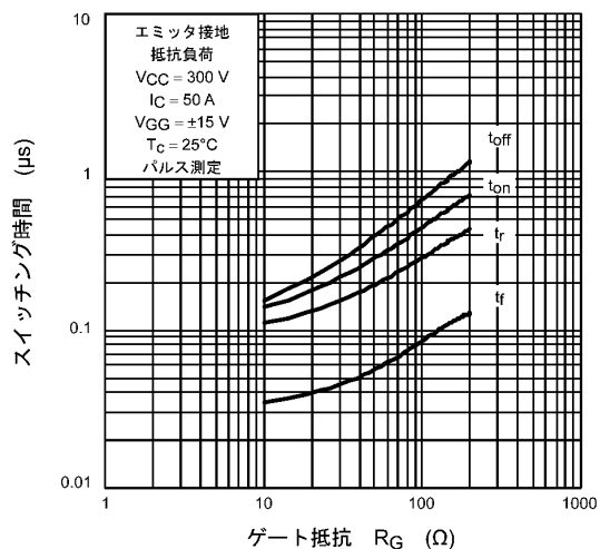
図 8.7 スwitchング時間 - R_G
