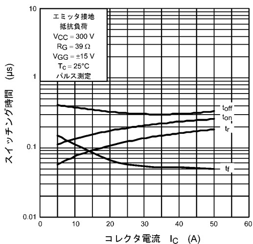
図 8.6 スイッチング時間 - I_C
