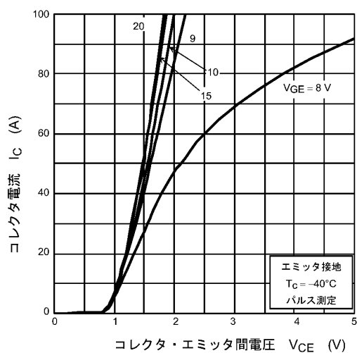
図 8.1 I_C - V_{CE}
