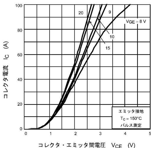
図 8.3 I_C - V_{CE}
