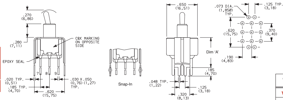
7301MD9__BE 3PDT
